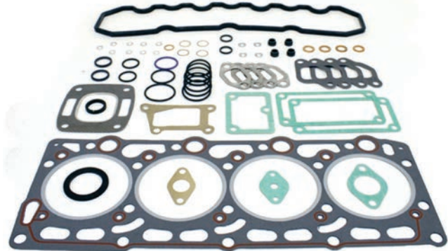
D30 AD30A, AQAD30A, MD30A TAMD30A, TMD30A
